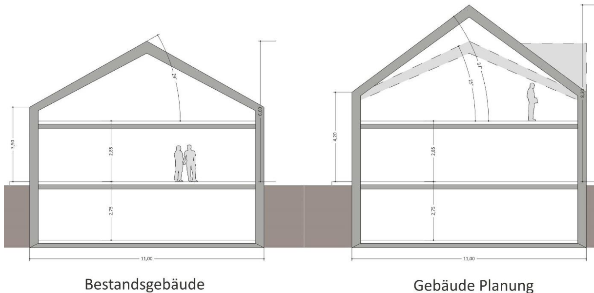
Abbildung 2: Gebäudeschnitte durch Bestandsgebäude (Mittelmaß aus bestehenden Gebäuden der Lindenstraße) und Gebäude Planung (schematische Darstellung)
